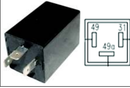
VF 283 12 V 3 UC CARGO / MAGIRUS FLAŞÖR
