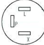
VF 501 12 V ELEKTROMEKANİK FLAŞÖR
