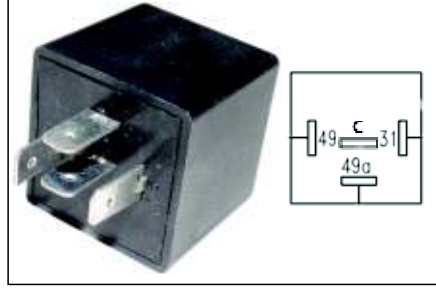
VF 277 12 V 4 UC KISA KANGOO / MEGANE AMPÜL HASSASİYET
