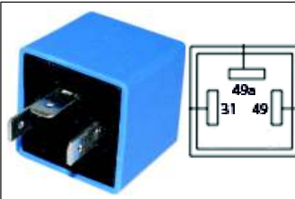
VF 290 12 V KISA FATİH / VW / SEAT / OPEL / ESCORT
