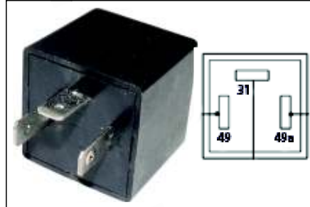
VF 288 12 V 3 UC TOFAŞ FLAŞÖR
