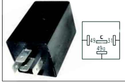
VF 286 12 V 4 UC RENAULT FLAŞÖR BRAKETSİZ
