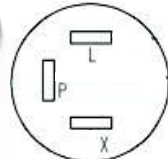
VF 502 24 V ELEKTROMEKANİK FLAŞÖR
