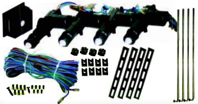
ZA4S MERKEZİ KİLİT SETİ - 4 KAPI - UZUN BOĞAZLI EXTRA
