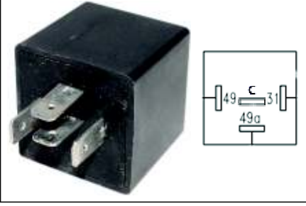
VF 276 12 V 4 UC RENAULT KANGOO FLAŞÖR
