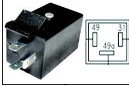
VF 284 12 V 3 P FORD FLAŞÖR KLİPSLİ
