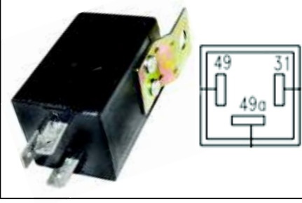
VF 285 24 V 3 UC CARGO MAGIRUS FLAŞÖR
