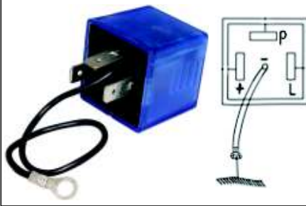
VF 012 12 V UNİVERSAL FLAŞÖR
